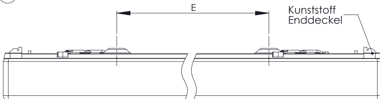
AOT-F: Grundblech ohne Kunststoff Enddeckel
